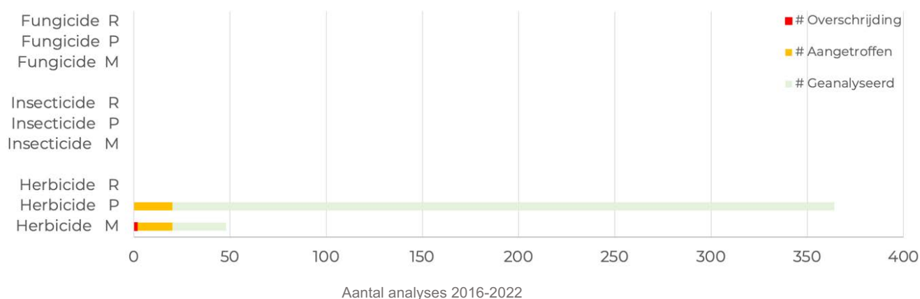
Figuur B9.3 Het aantal analyses met aangetroffen stoffen per type in het ruwwater (R), de pompputten (P) en het meetnet (M) in GWBG Edese bos (Ede).
