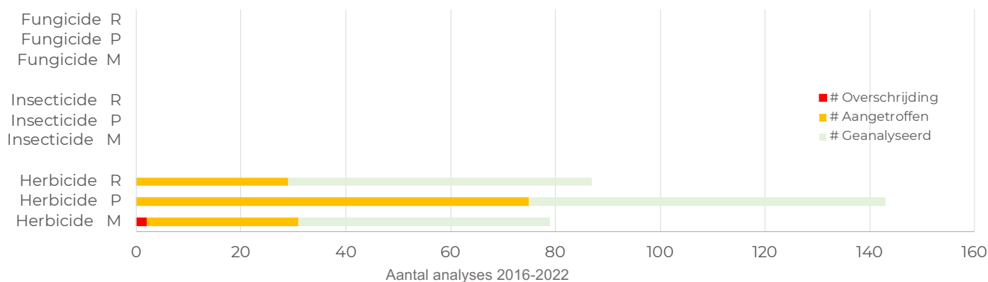
Figuur B27.3 Het aantal analyses met aangetroffen stoffen per type in het ruwwater (R), de pompputten (P) en het meetnet (M) in GWBG Velddriel.
