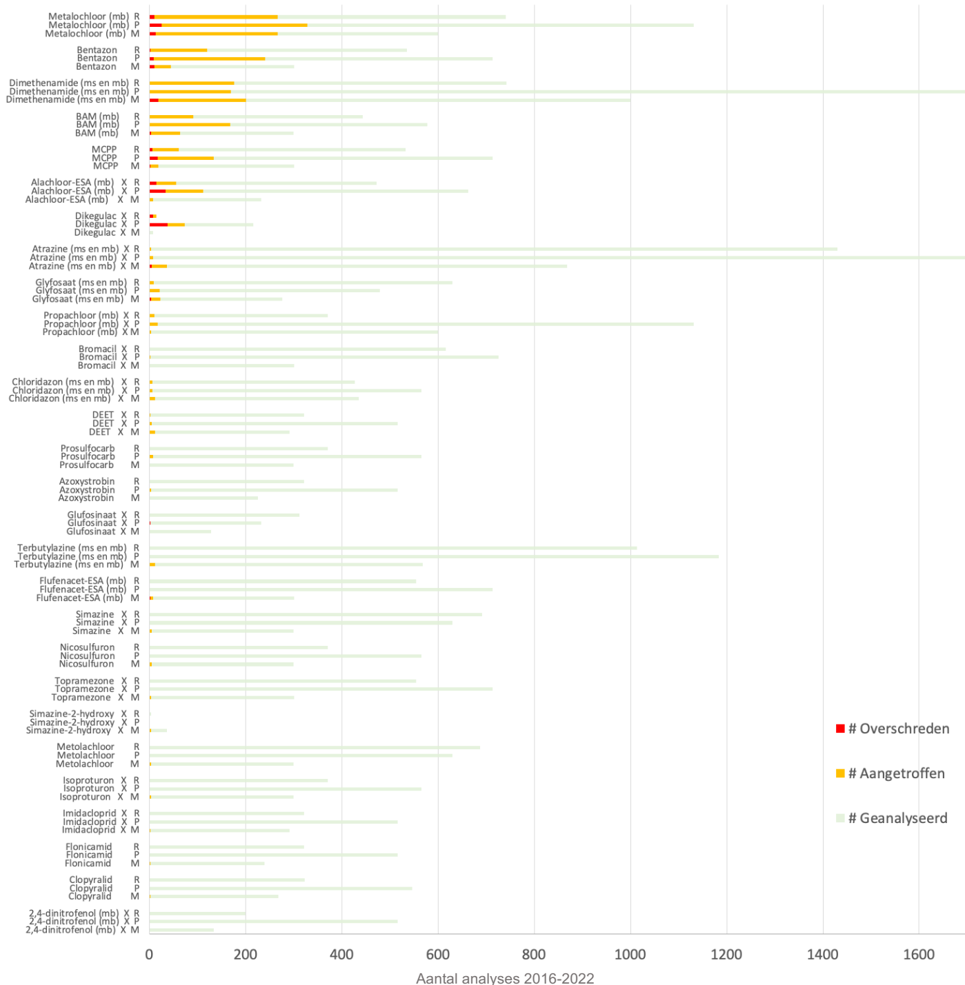
Figuur 4.5. Overzicht van aangetroffen stoffen in alle geanalyseerde monsters tussen 2016 en 2022, het aantal keer dat op de stof is geanalyseerd, het aantal keer dat de stof is aangetroffen en het aantal keer dat de concentratie de norm overschreed. Moederstoffen (ms) en metabolieten (mb) zijn samengenomen. Moederstoffen en humaan-toxicologisch relevante metabolieten zijn getoetst aan de norm van 0,1 µg/l, overige metabolieten zijn getoetst aan de norm van 1,0 µg/l. X= stof is niet meer toegelaten in de landbouw, R=ruwwater, P=pompputten, M=meetnet.
