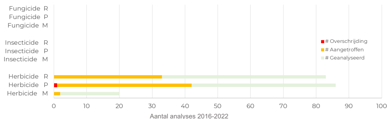
Figuur B20.3 Het aantal analyses met aangetroffen stoffen per type in het ruwwater (R), de pompputten (P) en het meetnet (M) in GWBG Lochem.
