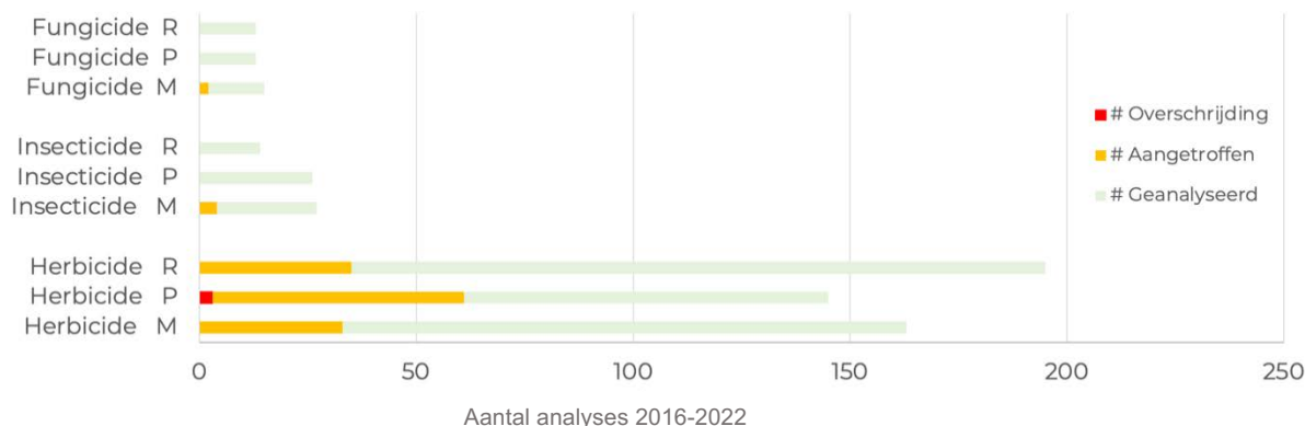
Figuur B3.3 Het aantal monsters met aangetroffen stoffen per type in het ruwwater (R), de pompputten (P) en het meetnet (M) in GWBG Corle (Winterswijk).
