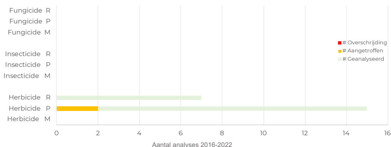
Figuur B29.3 Het aantal analyses met aangetroffen stoffen per type in het ruwwater (R), de pompputten (P) en het meetnet (M) in waterwingebied Wageningse Berg.
