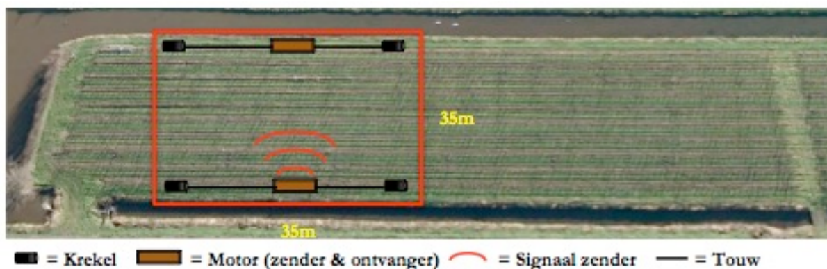
Figuur 1. Schematische weergave van een compleet krekelsysteem in een plot van 35x35 meter. Bestaande uit vier krekels en twee elektromotoren waarvan (één met zender en de andere met een ontvanger).
